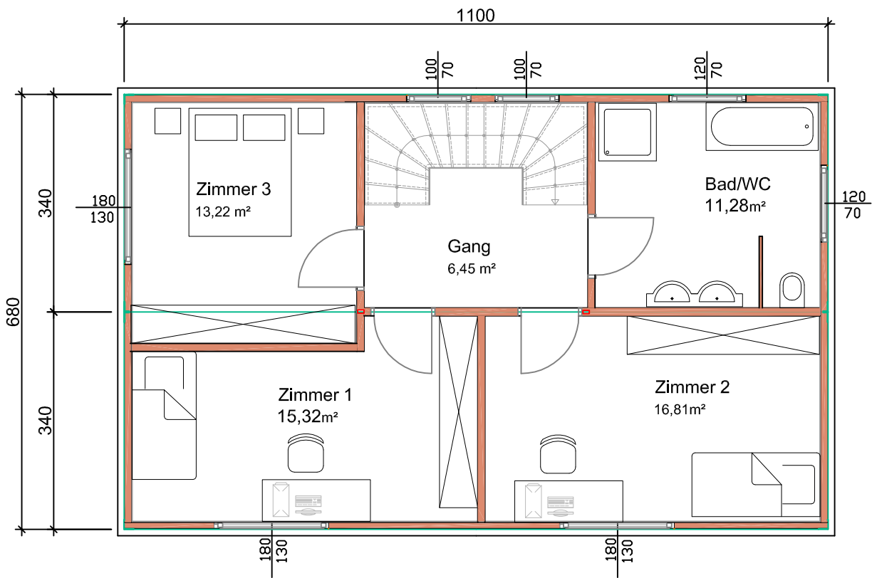
Obergeschoss WNFL 63,08 m 2
