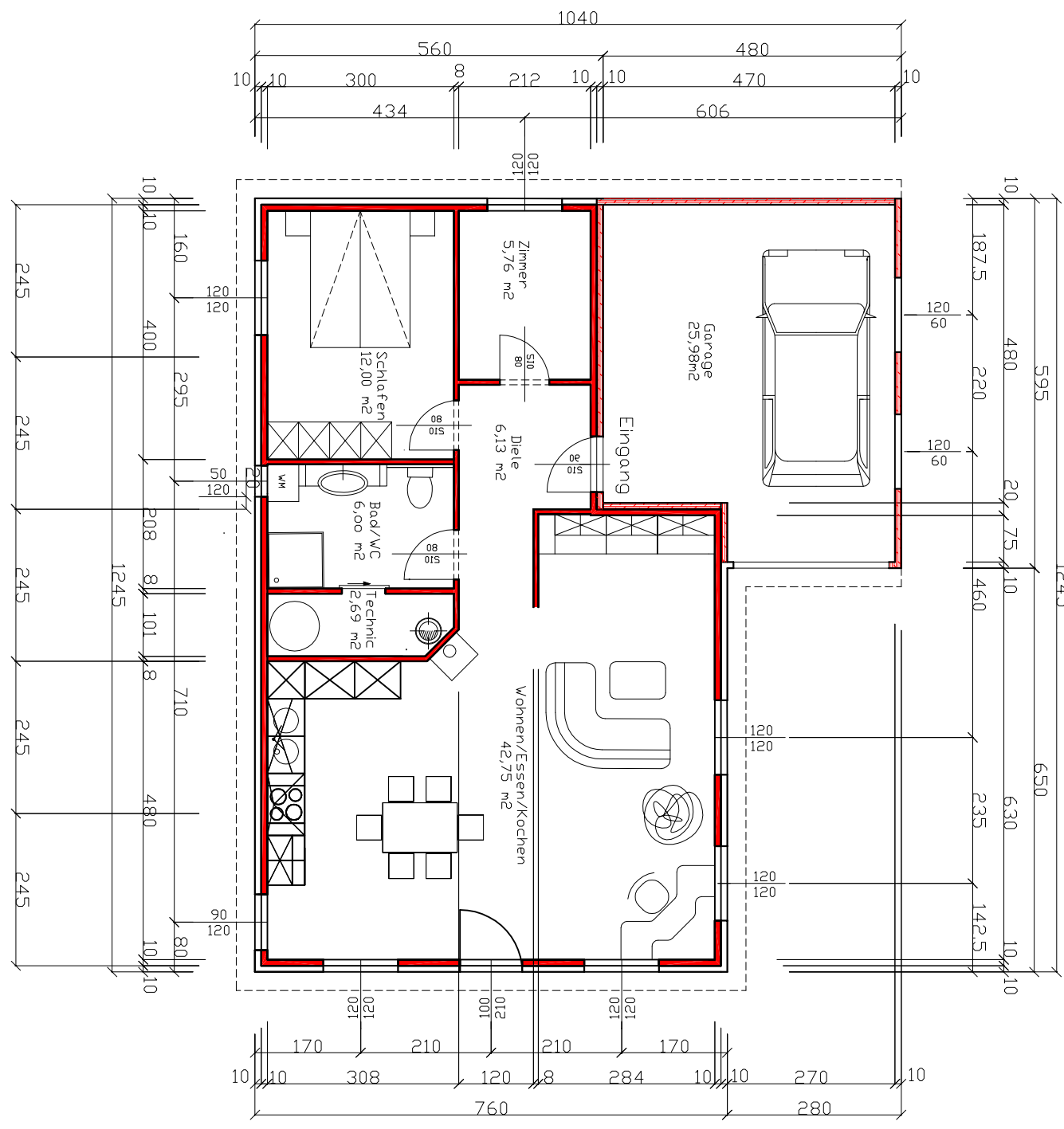
Erdgeschoss M 1:100
